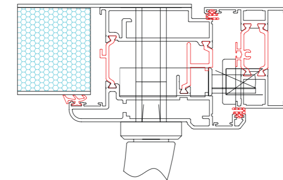
Jamb Detail
