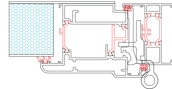
Jamb Detail
